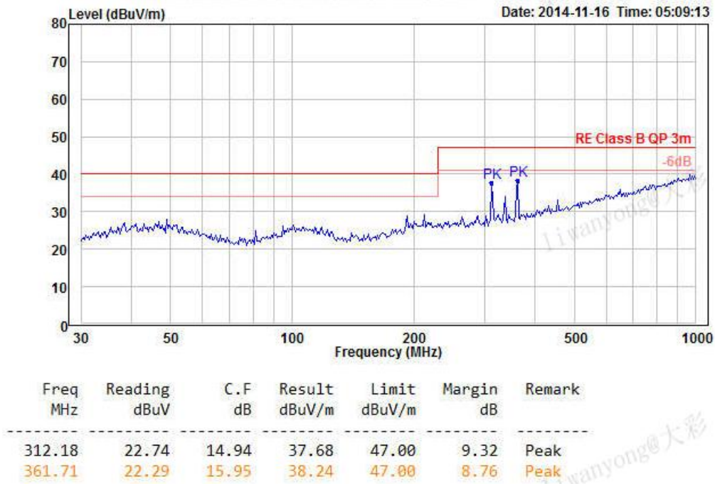
图 4-5 RE 测试水平方向
