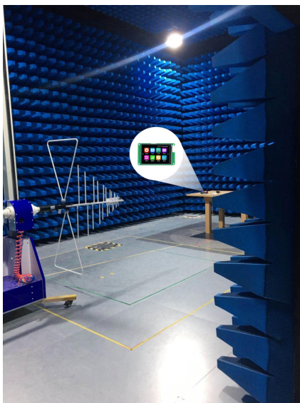
图 4-4 RE 测试图
