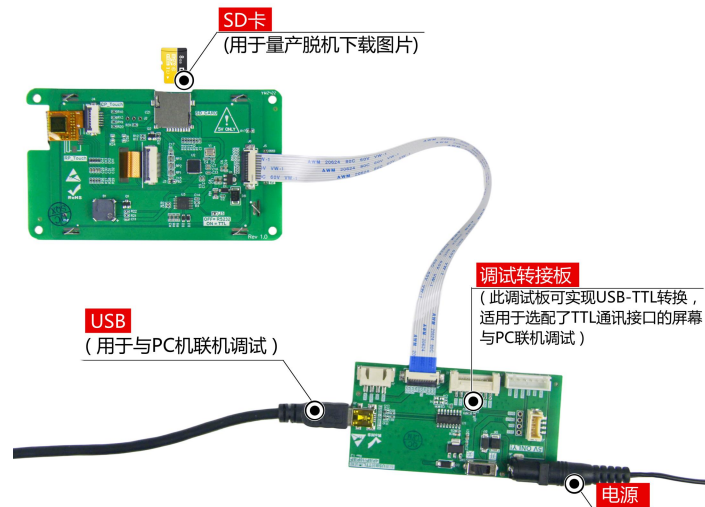
图 1-5 调试工具图
