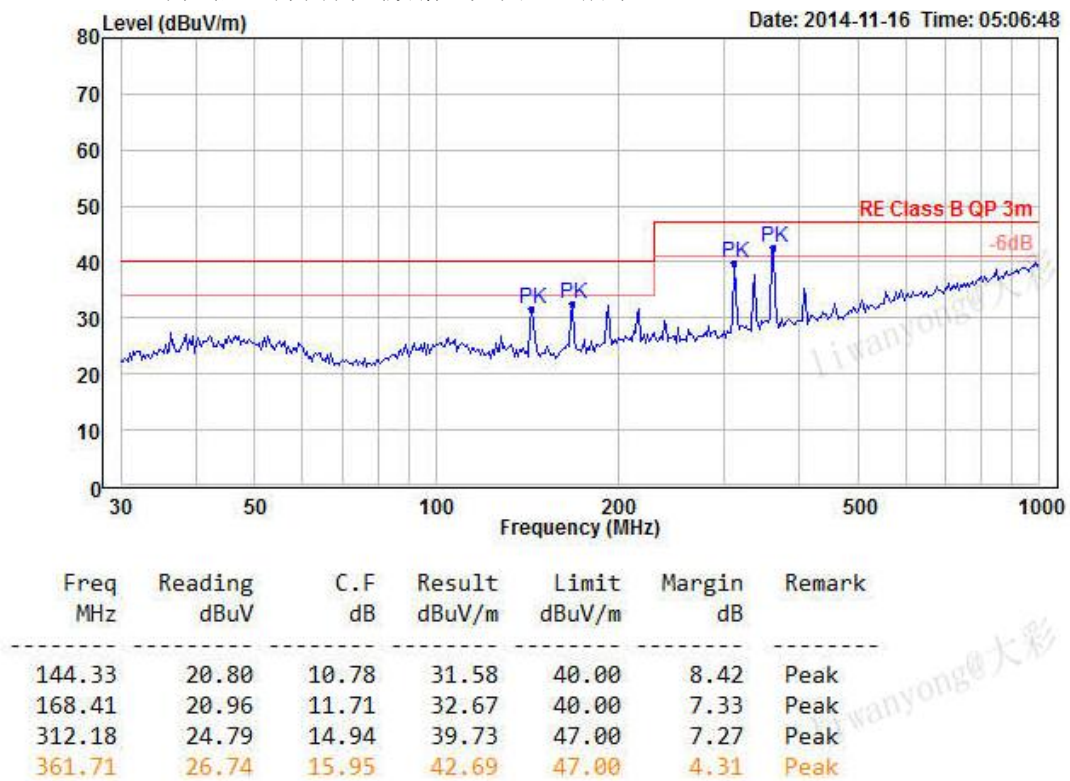
图 4-6 RE 测试垂直方向
